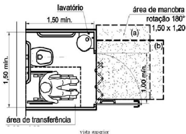
Figura 126 — Exemplo de cabine para sanita — Reformas — Área de manobra externa
