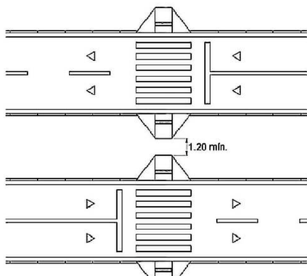
Figura 106 — Canteiro divisor de faixas - Exemplo 1
