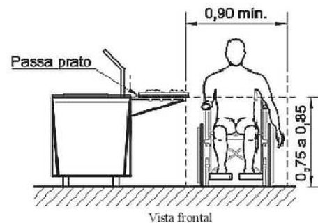
Figura 164 — Auto-atendimento em refeitórios — Exemplo
