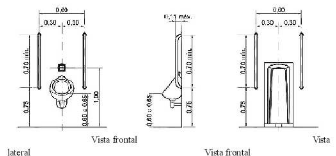
Figura 140 — Mictórios — Exemplos
