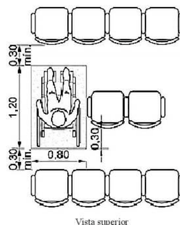
Figura 151 — Espaços para P.C.R. em fileira intermediária — Exemplo
