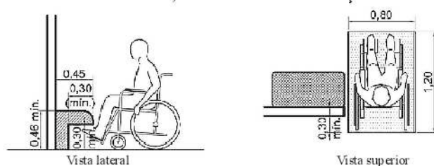
Figura 144 — Bancos para vestiários
