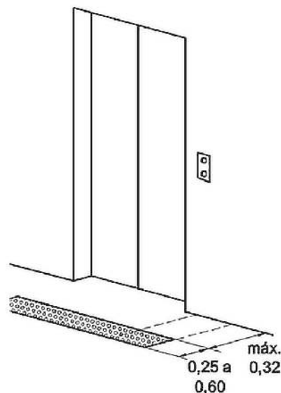
Figura 64 — Exemplo de sinalização táctil de alerta junto à porta de elevador
