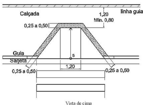
Figura 62 — Exemplo de sinalização táctil de alerta nos rebaixamentos das calçadas
