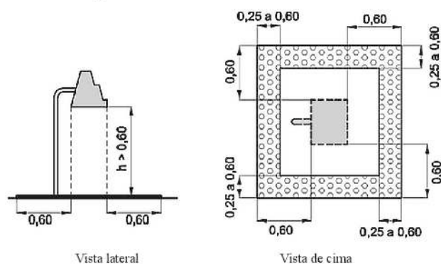
Figura 60 — Sinalização táctil de alerta em obstáculos suspensos — Exemplo
