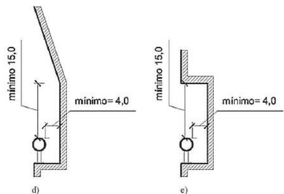
Figura 15 — Empunhaduras (dimensões em centímetros)
