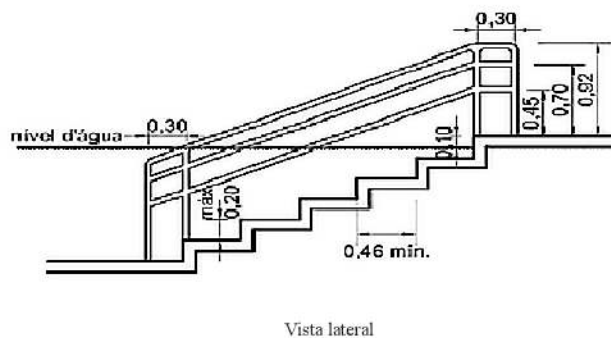
Figura 156 — Escada submersa — Exemplo
