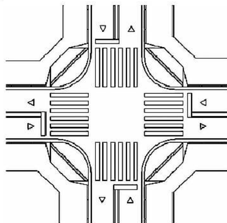
Figura 102 – Esquina – Rebaixamento C
