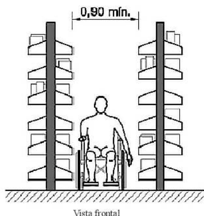
Figura 158 — Estantes em bibliotecas — Exemplo
