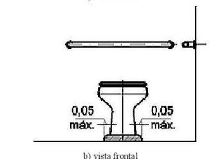
Figura 121 — Adequação de altura da sanita com sóculo.
