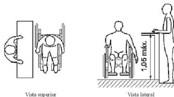
Figura 165 — Bilheteria — Exemplo
