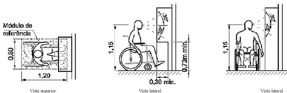
Figura 167 — Máquina de atendimento automático — Exemplo
