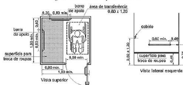
Figura 144 — Bancos para vestiários
