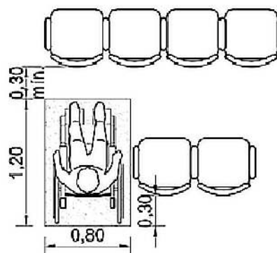
Figura 150 — Espaços para P.C.R. na segunda fileira
