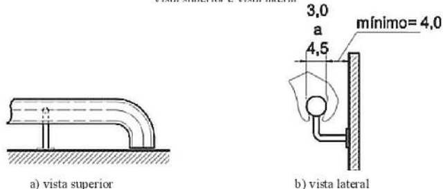
Figura 85 — Empunhadura de corrimão - Exemplo
