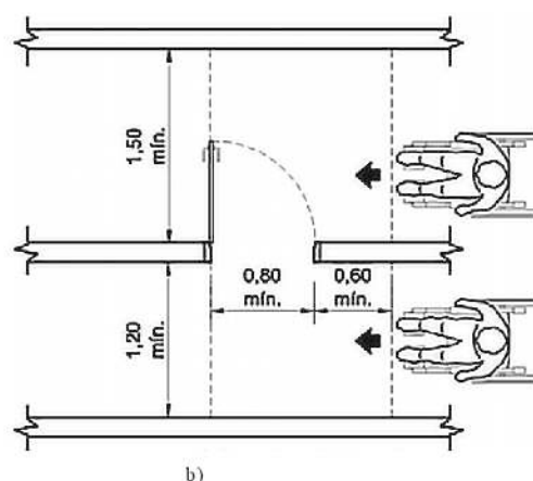
Figura 92 — Exemplo de aproximação de porta frontal
