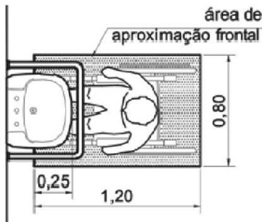
Figura 135 — Área de aproximação para P.C.R.
