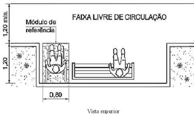
Figura 162 — Banco — Exemplo
