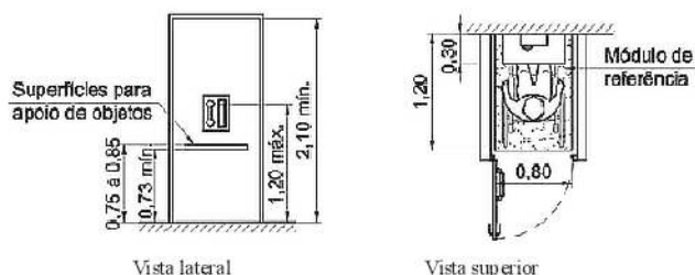
Figura 160 — Cabina telefónica — Exemplo
