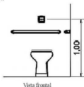
Figura 122 — Altura de accionamento da descarga
