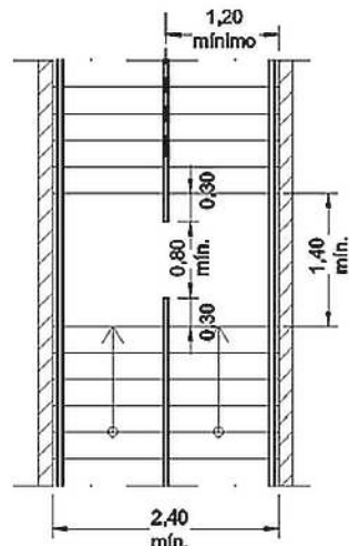
Figura 89 — Corrimão intermediário
