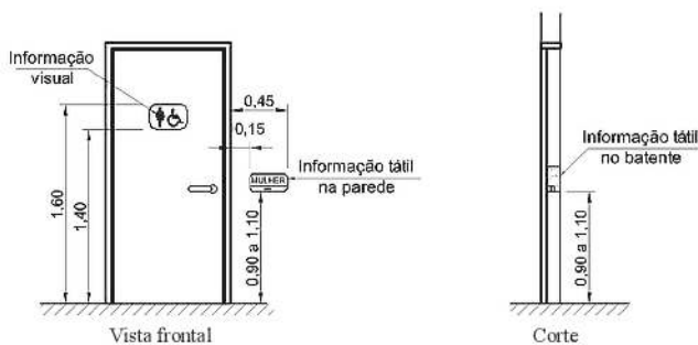
Figura 55 — Sinalização visual e tátil em portas – Exemplos
