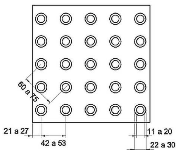
Figura 59 — Sinalização táctil de alerta — Modulação do piso (dimensões em milímetros).
