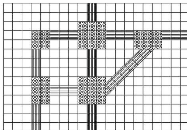
Figura 67 — Composição de sinalização tátil de alerta e direccional — Exemplo
