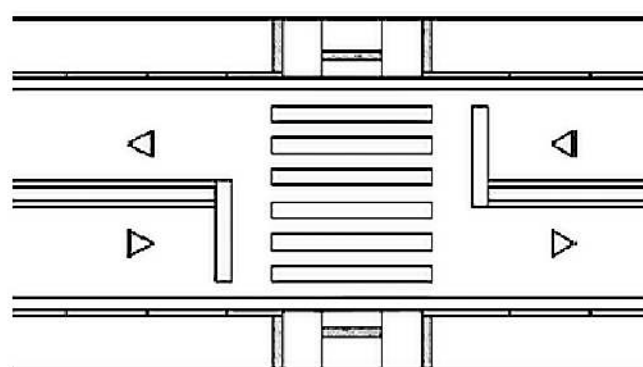
Figura 105 — Meio da faixa – Rebaixamento C
