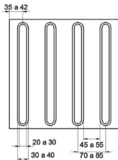
Figura 66 — Sinalização tátil direccional — Modulação do piso (dimensões em milímetros)
