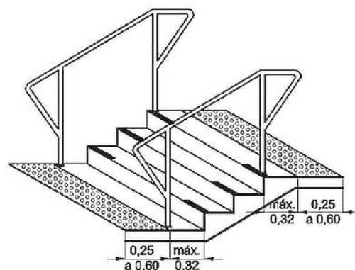
Figura 63 — Exemplo de sinalização táctil de alerta nas escadas
