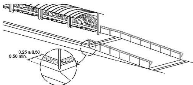
Figura 65 — Exemplo de sinalização tátil de alerta junto a desnível em plataforma de embarque e desembarque
