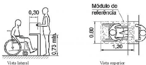
Figura 163 — Balcão — Exemplo
