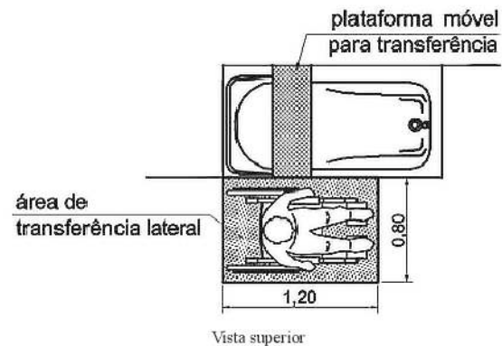
Figura 132 — Plataforma móvel para transferência
