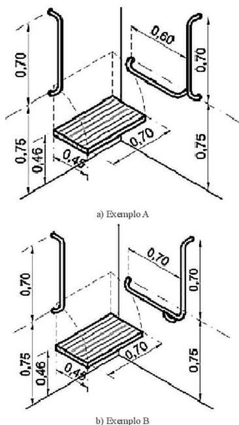
Figura 130 — Perspectiva da cabine com as barras de apoio
