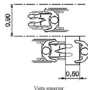
Figura 166 — Balcão de atendimento — Exemplo
