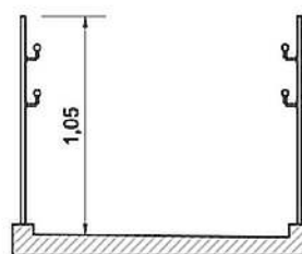
Figura 90 — Exemplo de guarda-corpo
