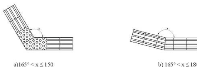
Figura 68 — Composição de sinalização tátil de alerta e direccional — Exemplos de mudanças de direcção
