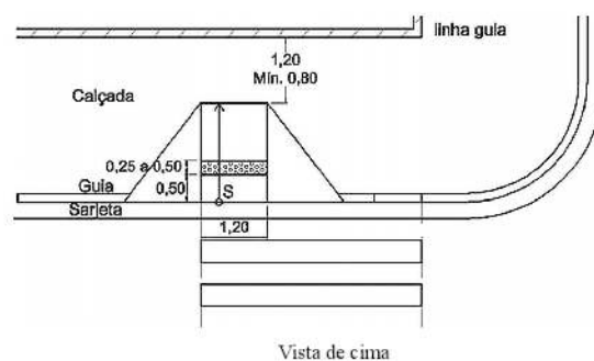
Figura 61 — Exemplo de sinalização táctil de alerta nos rebaixamentos das calçadas
